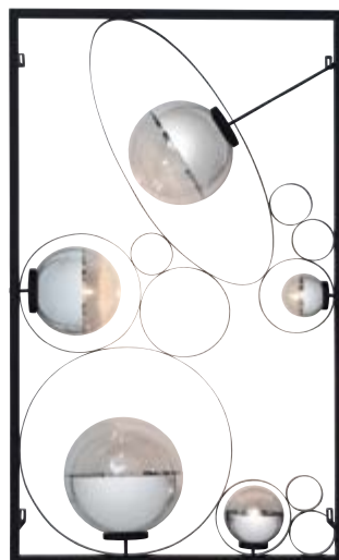
39047 2xE14/LED 4W 3xE27/LED 8W 191x105x50 EEI:A
